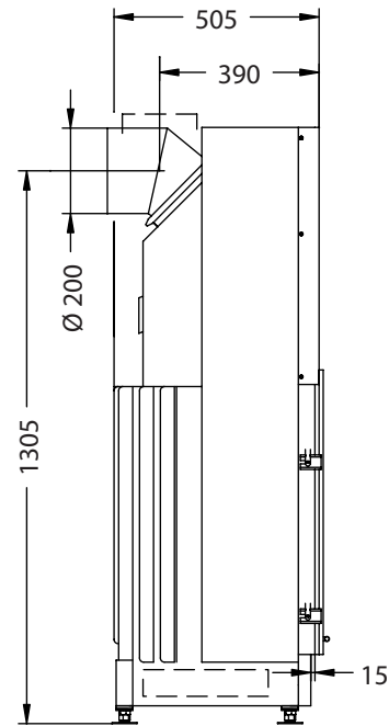
Seitenansicht M~1:20
