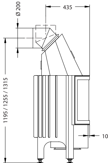
Seitenansicht M~1:20
