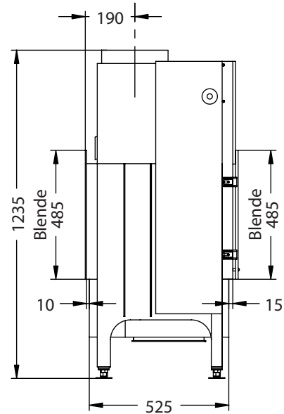
Seitenansicht M~1:20
