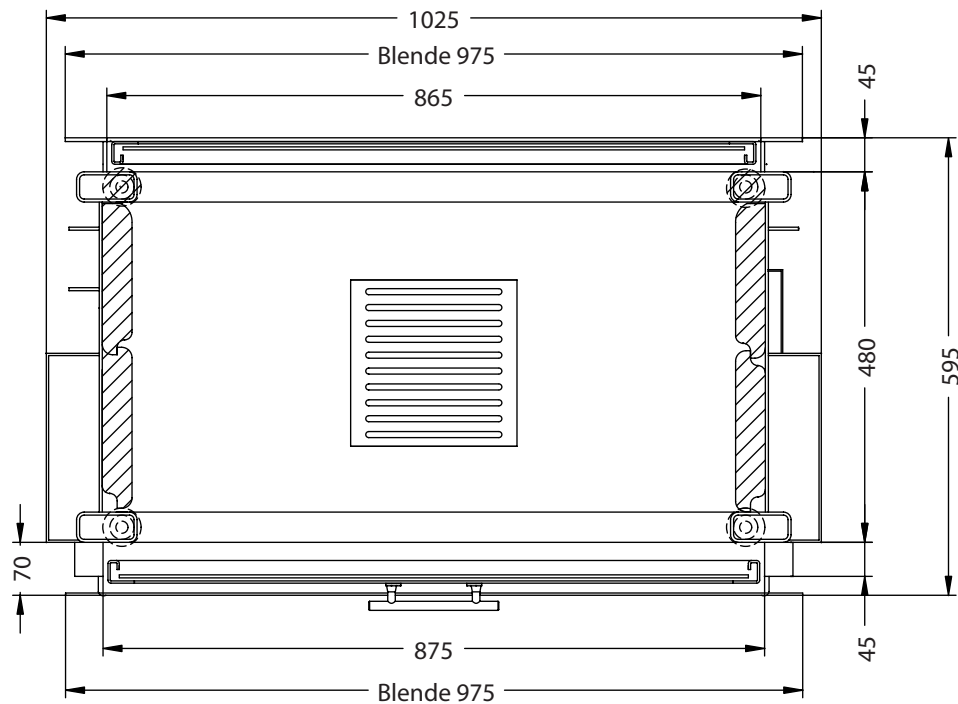
Horizontalschnitt M~1:10
