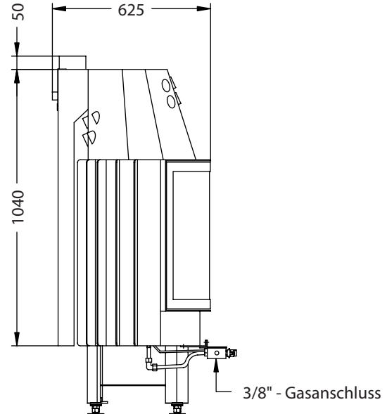
Seitenansicht M~1:20
