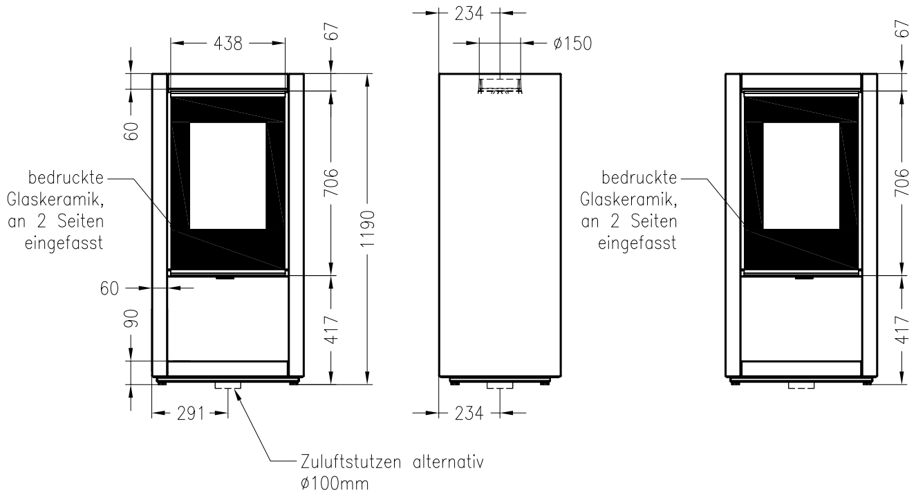
Vorderansicht M ~1:20
