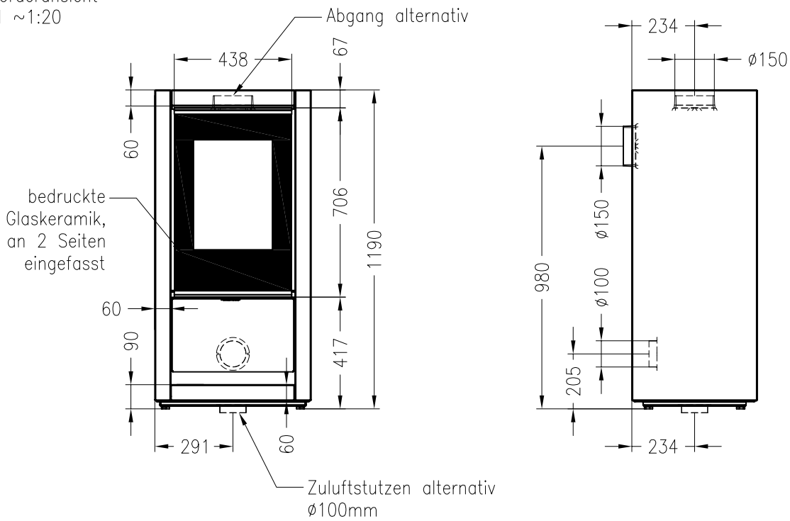
Seitenansicht M ~1:20
