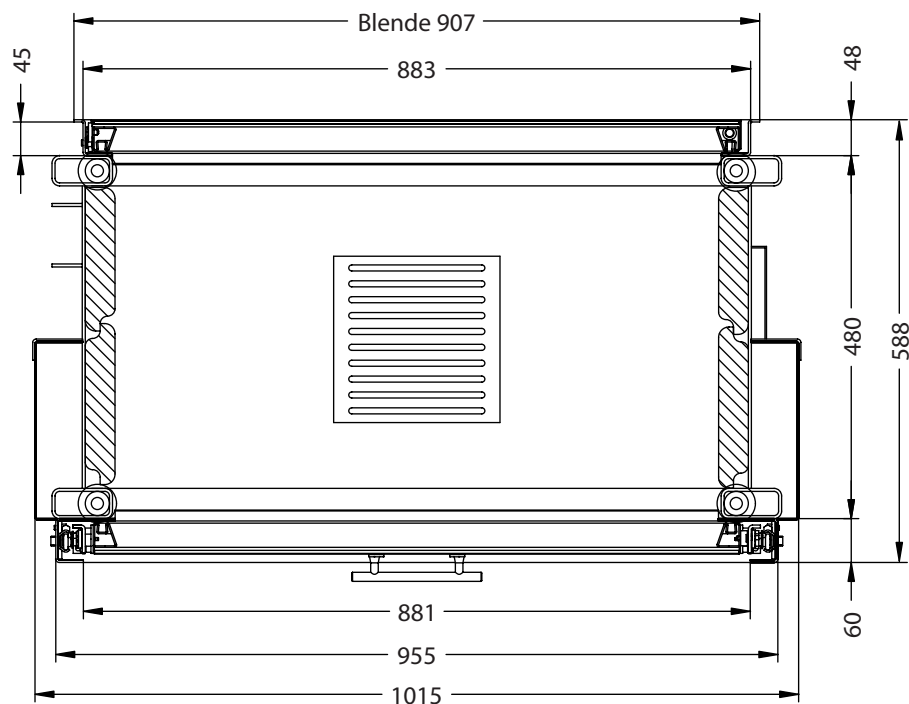
Horizontalschnitt M~1:10
