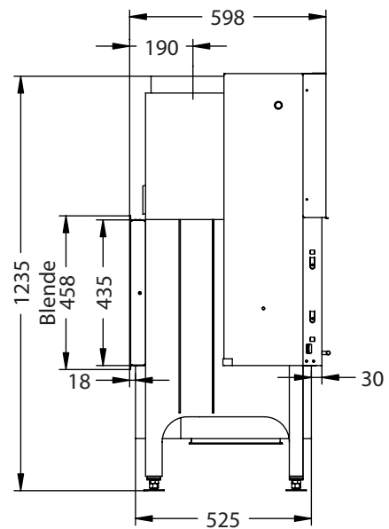
Seitenansicht M~1:20
