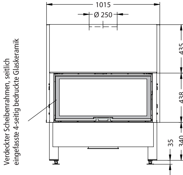
Vorderansicht M~1:20
