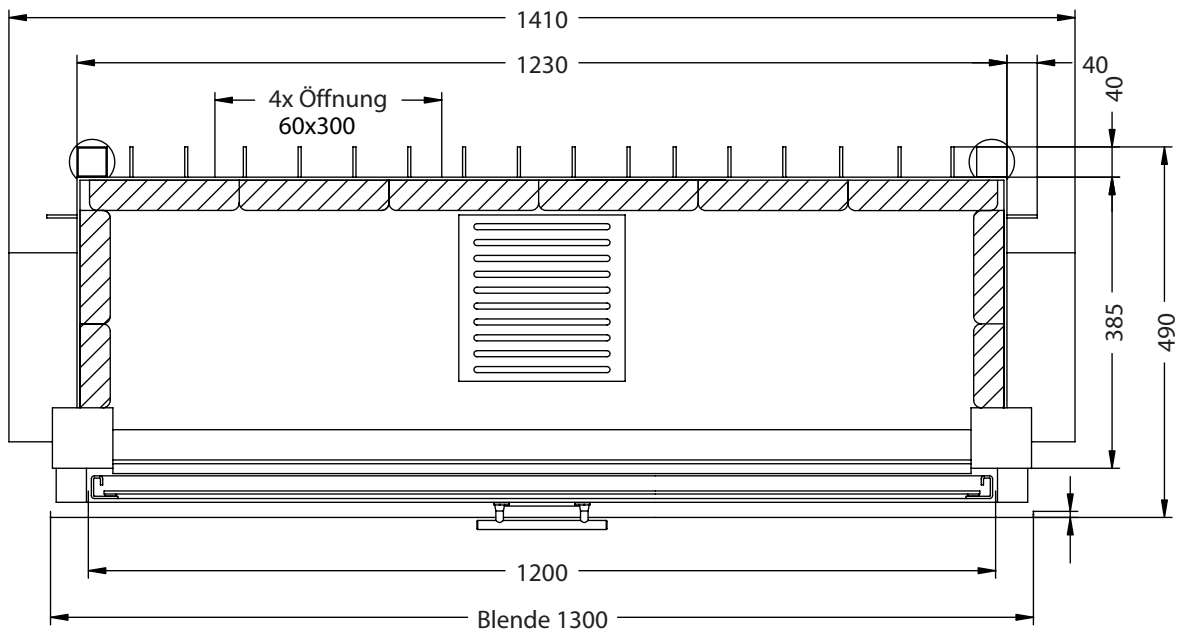
Horizontalschnitt M~1:10
