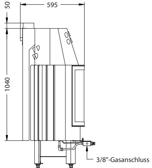
Seitenansicht M~1:20
